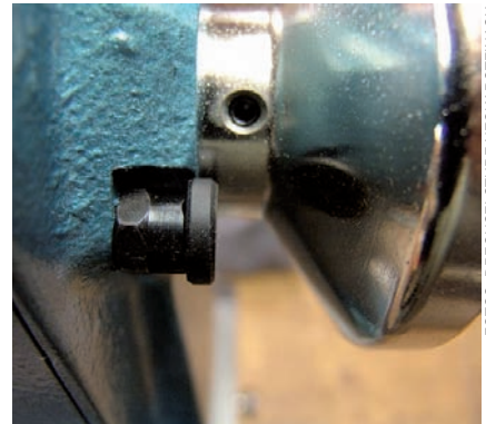
Die Arretierung der Spindel besitzt jetzt keinen Federstift mehr, sondern kann nun fest in der Teilscheibe arretiert werden.
